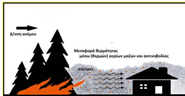
Σχέδιο 4. Τρόποι ροής της θερμότητας σε μια δασική πυρκαγιά, που εξελίσσεται πλησίον κτιρίου και απεικόνιση πιθανού τρόπου μετάδοσης δασικής πυρκαγιάς με μεταφερόμενες καύτρες σε κτίρια παρουσία ισχυρού ανέμου
